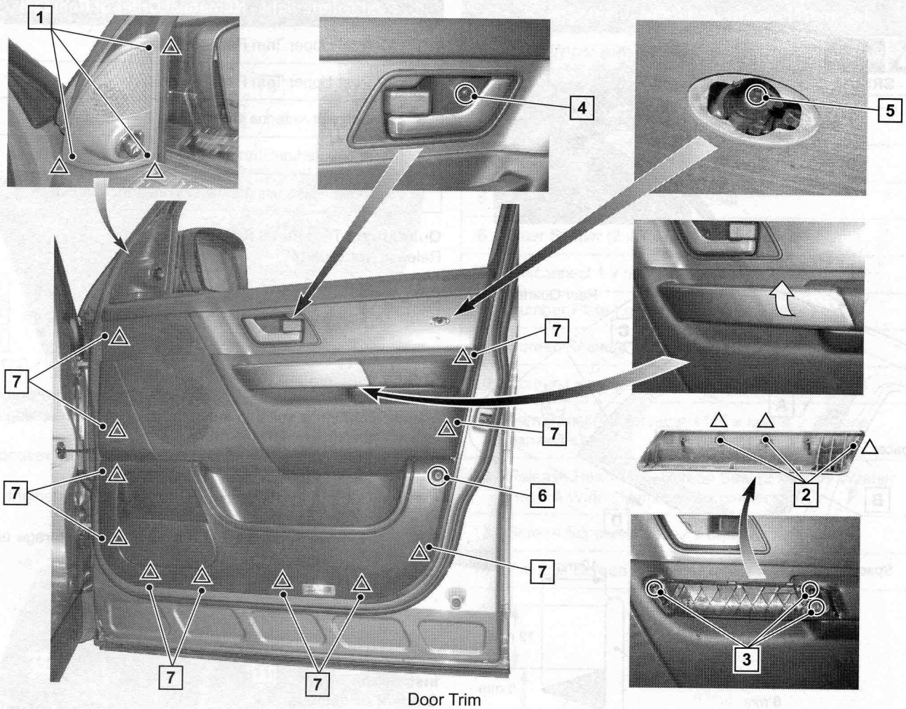
Door Trim
